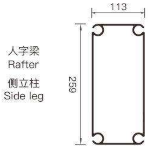
框架规格 Specification
