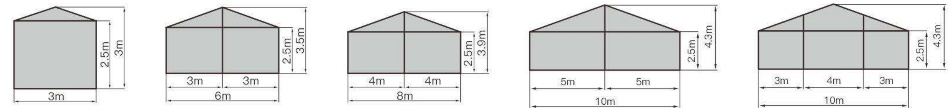
框架规格 Specification
